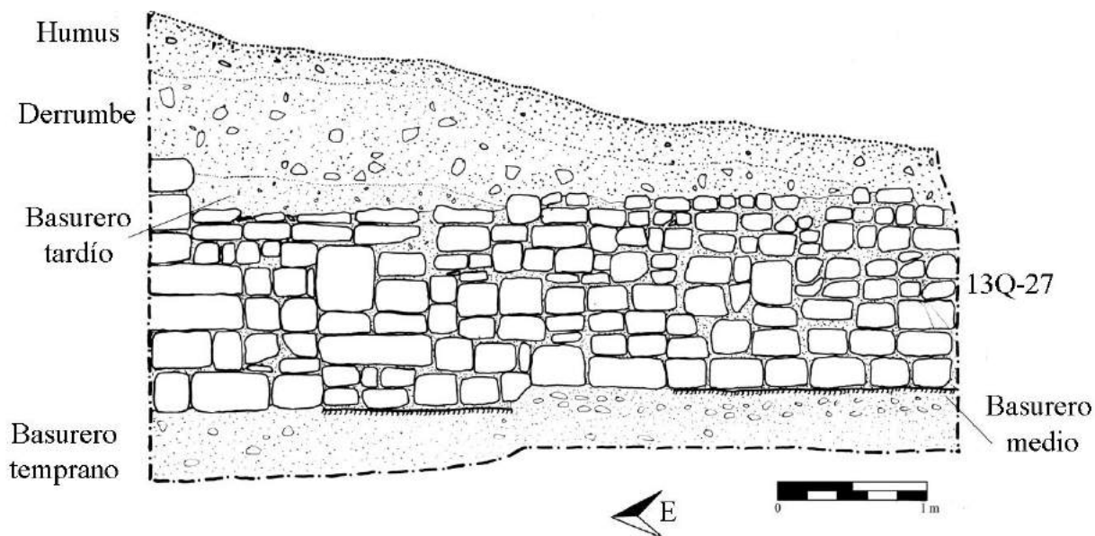
Figura 5.20 Perfil sur de la Unidad CR22-4, fachada de la Estructura 13Q-27 (Dibujo por P. Castillo, digitalización de A. Coronado y R. Morales Forte).
