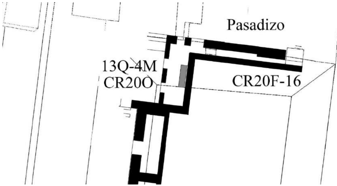
Figura 3.6. Planta final de la Operación CR200 (Dibujo por E. Bustamante).
