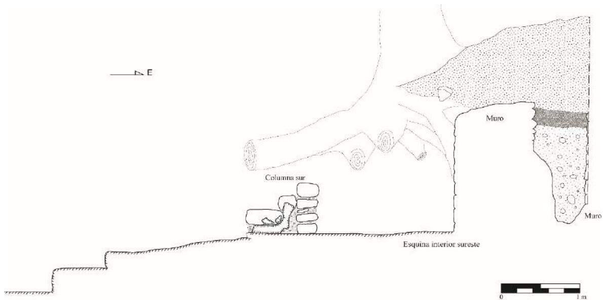
Figura 9.19. Corte este-oeste de la Estructura 13R-45, que muestra los dos escalones de acceso, la columna sur con restos de estuco, y los muros adyacentes que limitan la estructura en su lado este (Dibujo P. Castillo y digitalización A. Cajas).
