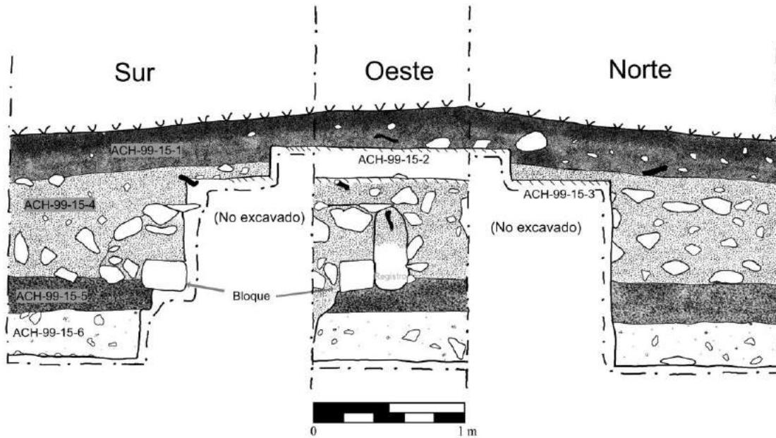
Figura 13.51 Perfiles de la Unidad ACH99-15 (Dibujo por L. Auld-Thomas).
