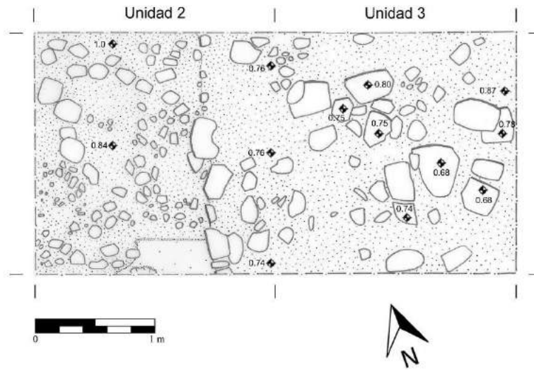
Figura 12.10 Planta de las unidades ACH 2 y 3 al remover el lote 3 (Dibujo por E. Arredondo).
