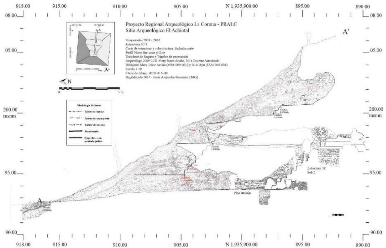
Figura 1.19 Perfil este de la Estructura 5C-01 (Dibujo por J. Ajin/ M. Acuña; digitalizado por J. González).
