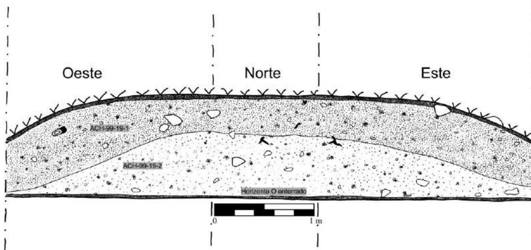
Figura 13.59 Perfil Oeste-Noreste de la Unidad ACH-99-19 (Dibujo por L. Auld-Thomas)
