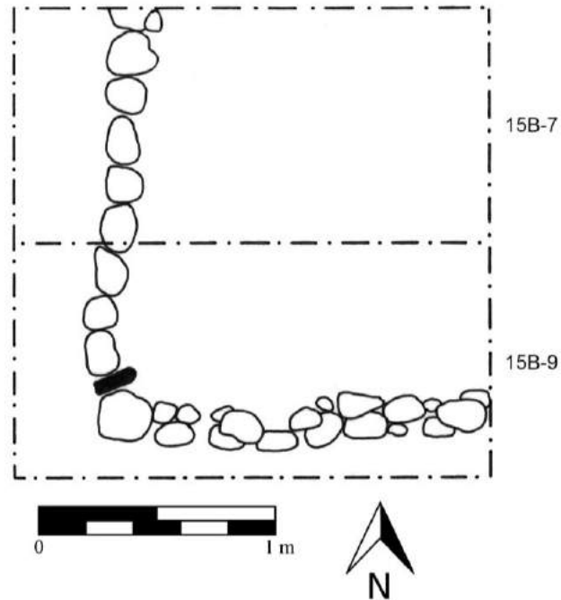
Figura 10.16 Planta de las unidades CAR15B-7 y CAR15B-9 (Dibujo por D. Chatelain).
