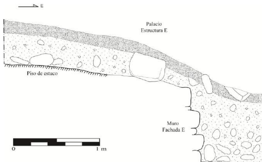
Figura 4.10 Fachada este de Estructura 13Q-4E, registrada en CR-20EC-15 (Dibujo y digitalización por A. Cajas).
