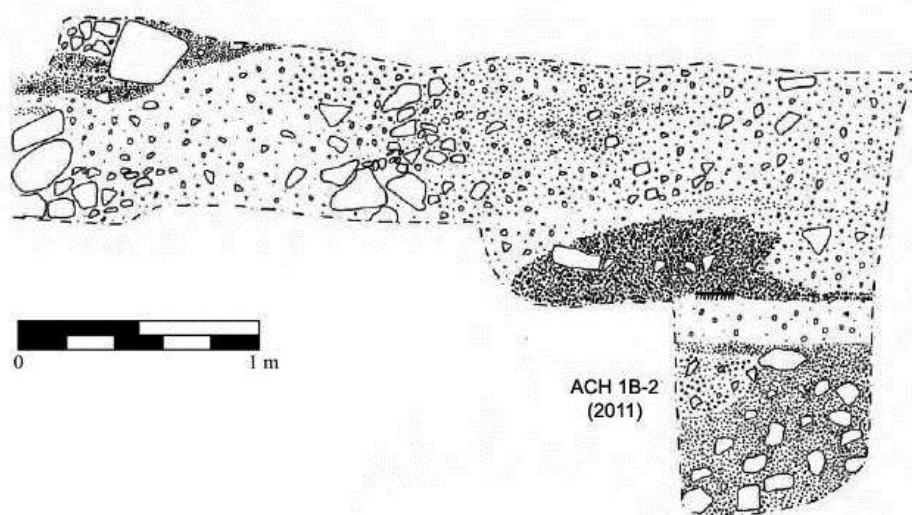
Figura 14.9 Perfil norte del Túnel 11 (modificado de Acuña 2013: fig. 5.46)
