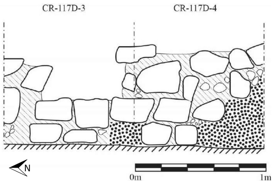
Figura 9.4 Elevación del muro interno en la Estructura 13R-7 (Dibujo por J. A. González)
