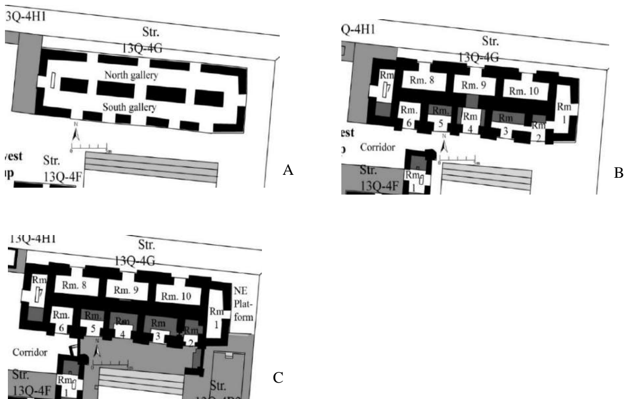
Figura 5.7 Evolución arquitectónica de 13Q-4G. A Fase Halcón A; B Fase Halcón B; C Fase Tucán (Dibujos por M. Lamoureux-St-Hilaire 2018 Fig. 5.21, 5.47, 5.49: 126, 155, 160).
