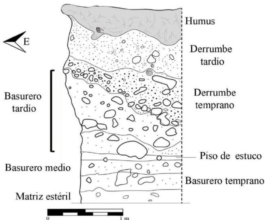
Figura 5.18 Perfil oeste de la Unidad CR22-5 (Dibujo por R. Morales Forte).
