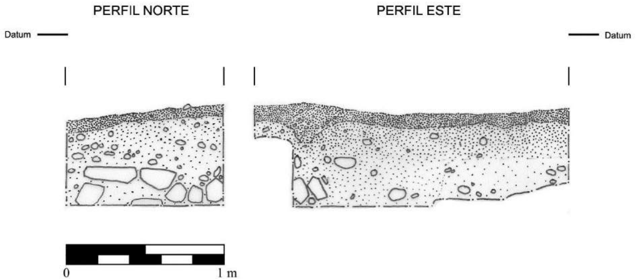
Figura 12.5 Perfiles norte y este de la Unidad ACH 3C-1 (dibujo por E. Arredondo).
