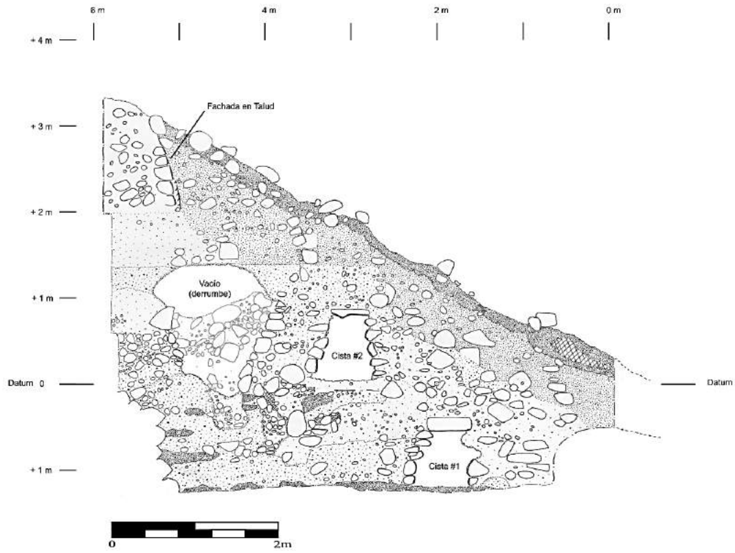
Figura 12.19 Perfil sur del Saqueo 2 (Dibujo por E. Arredondo).
