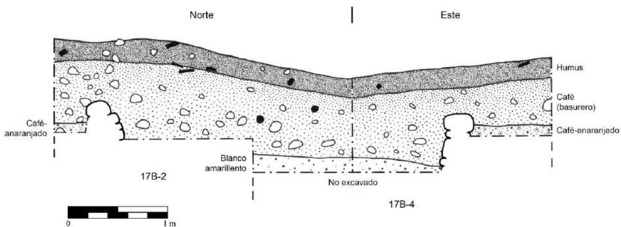
Figura 10.28 Perfil de las Unidades CAR17B-2 y Car17B-4 (Dibujo por D. Chatelain).
