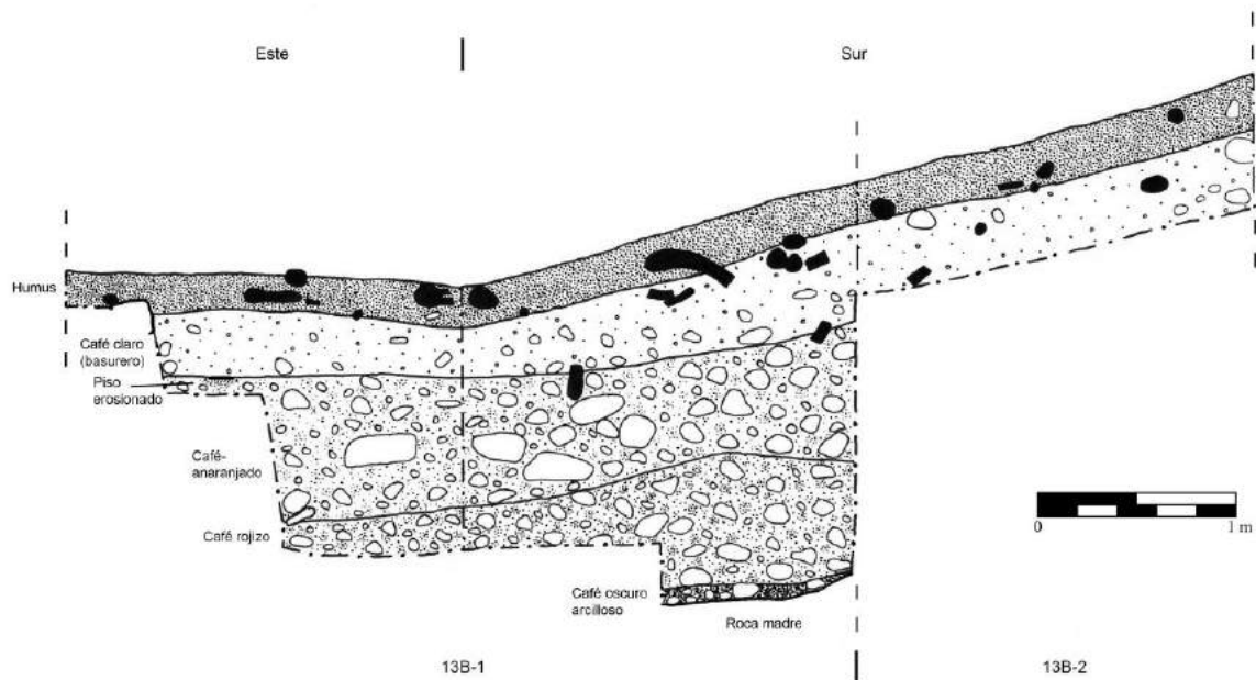
Figura 10.4 Perfiles de las unidades CAR13B-1 y CAR13B-3 (Dibujo por D. Chatelain).
