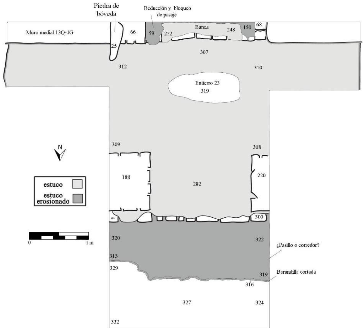
Figura 5.6 Cuarto 9 de la Estructura 13Q-4G, unidades CR20G-15, CR21N-2 y CR21N-7 (Dibujo por R. Morales Forte).
