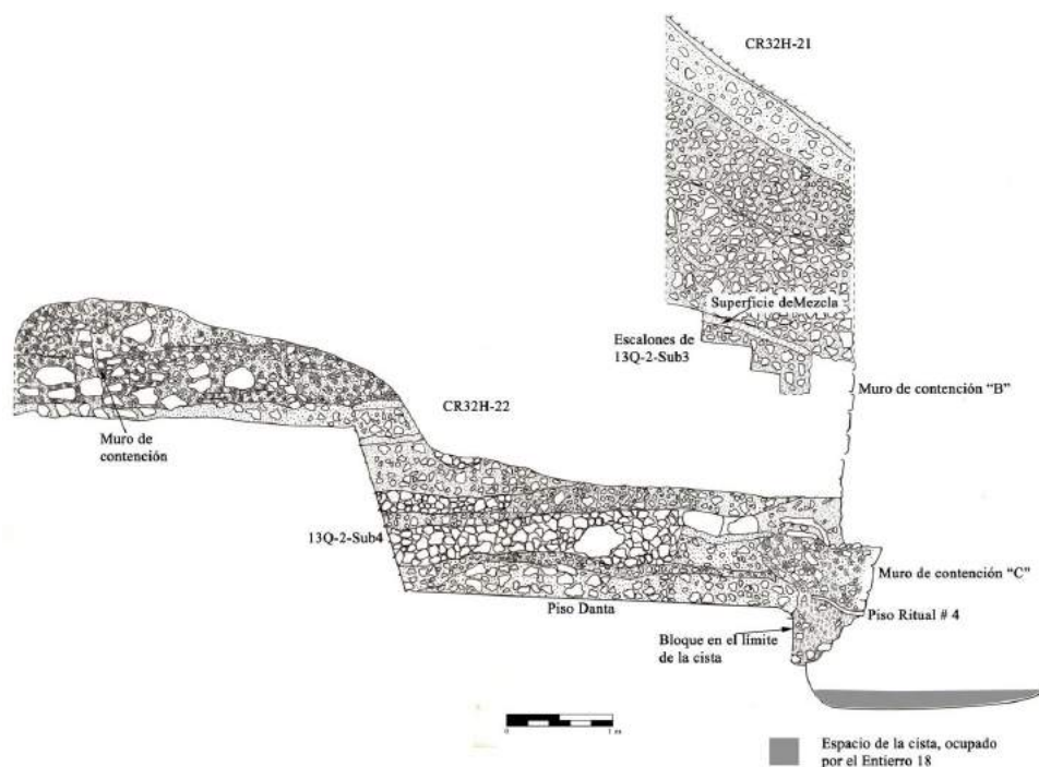
Figura 1.12 Perfil que muestra los restos de la Subestructura 13Q-2-Sub4, descubierto en 2015 (Dibujo por E. Gómez).
