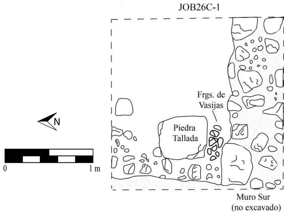
Figura 11.21 Planta de rasgos de la parte superior de la Estructura 7M-1 (Dibujo por J. Ponce)
