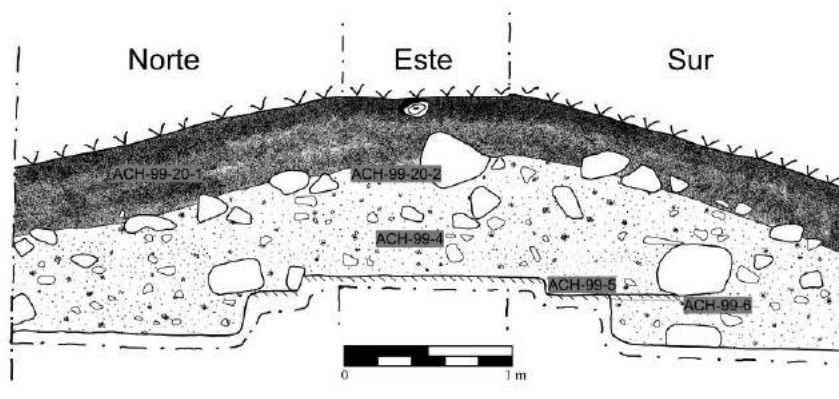
Figura 13.56. Perfiles de la Unidad ACH99-20 (Dibujo por L. Auld-Thomas).
