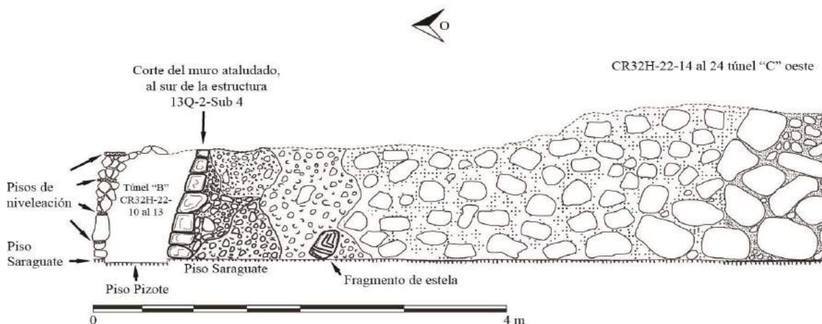
Figura 20.6 Perfil sur del túnel en el eje central de la Estructura 13Q-2 (Dibujo por Rony López)
