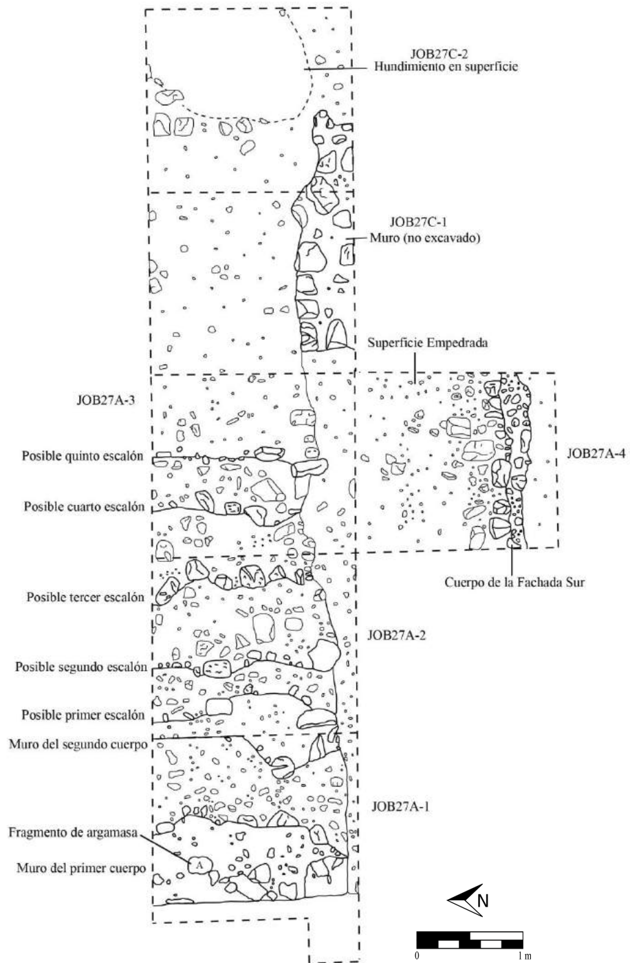
Figura 11.27 Planta de rasgos arquitectónicos superficiales en la Estructura 7M-2 (Dibujo por J. Ponce)
