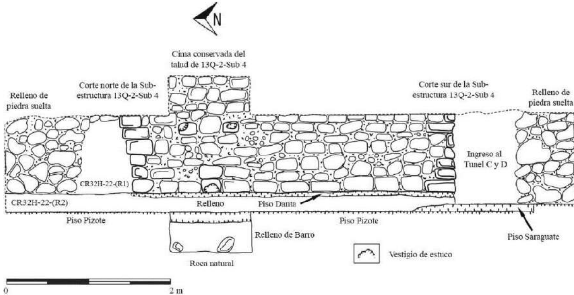
Figura 6.6 Vista de la fachada conservada de la Estructura 13Q-2-Sub 4, descubierta por los túneles A y B, y en el registro CR32H22-R2 (Dibujo por R. López).
