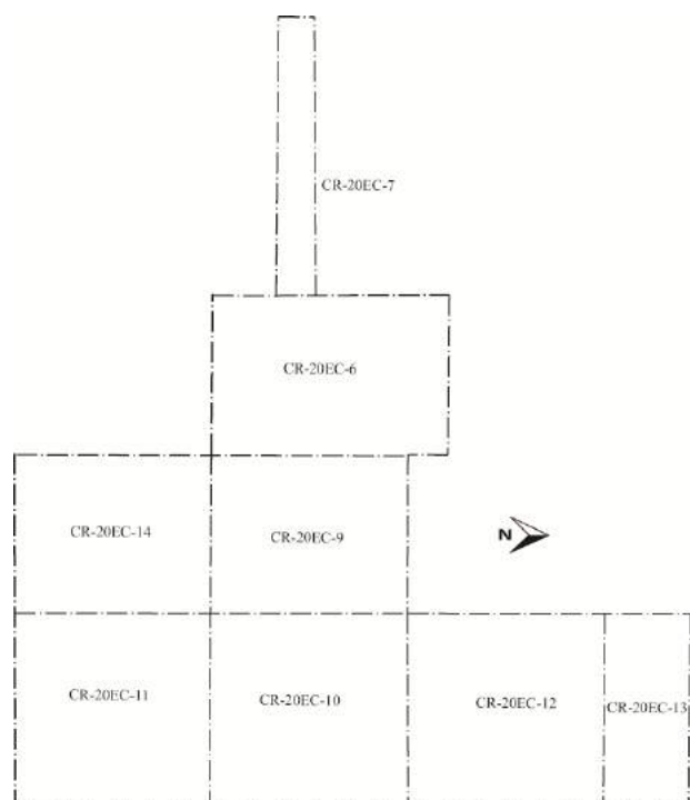
Figura 4.2 Croquis de unidades en la Estructura 13Q-4E, Operación CR-20EC (Digitalización por A. Cajas).
