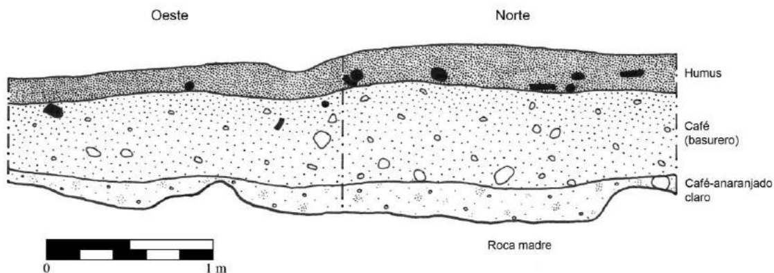
Figura 10.14 Perfil de la Unidad CAR15B-5 (Dibujo por D. Chatelain).
