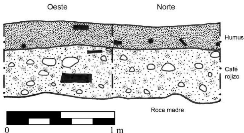
Figura 10.32 Perfil de la Unidad CAR18A-1 (Dibujo por D. Chatelain).
