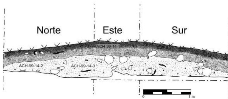
Figura 13.48 Perfil Norte-Este-Sur de la Unidad ACH-99-14 (Dibujo por L. Auld-Thomas)
