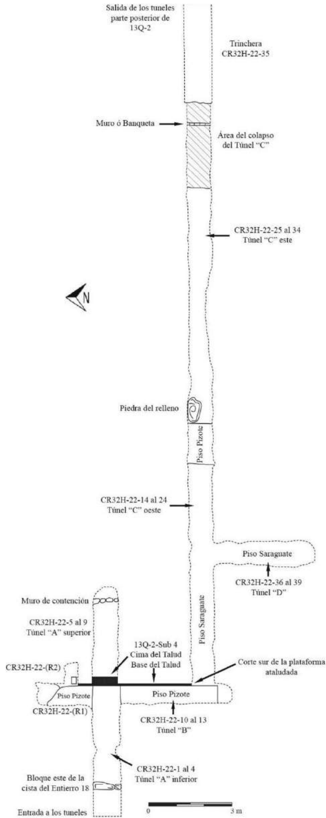
Figura 6.1 Planta general de las excavaciones en los túneles de la Estructura 13Q-2 (Dibujo por R. López).
