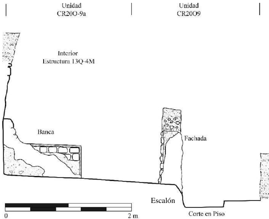
Figura 3.3. Corte E-O con vista al sur, mostrando el interior del cuarto, muro externo y parte de la banqueta frontal a la estructura (Dibujo por E. Bustamante)
