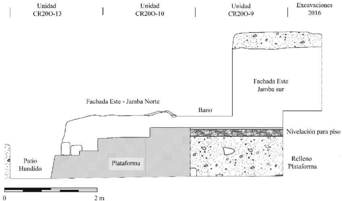
Figura 3.4. Perfil norte sur vista al este de las unidades CR200-9, -10, y -13. Se muestra fachada oeste de la Estructura 13Q-4M, así como los cuerpos de la plataforma de ésta (Dibujo por E. Bustamante).
