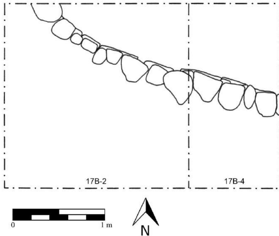
Figura 10.29. Planta de las unidades CAR17B-2 y CAR17B-4 (Dibujo por D. Chatelain)
