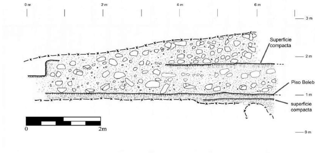
Figura 14.21 Perfil Este del Saqueo 2, Túnel Medio (ACH-TN3) (Dibujo por P. Castillo, calco por A. Coronado).
