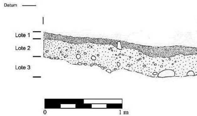
Figura 12.13 Perfil oeste de la Unidad ACH 3C-2 (Dibujo por E. Arredondo).
