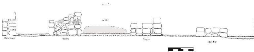
Figura 9.21 Corte longitudinal norte-sur de la Estructura 13R-45, con proyección de la ubicación del Altar 5 en su interior. (Dibujo por A. Cajas).
