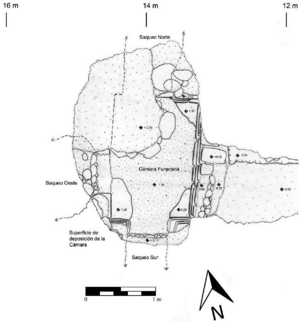
Figura 12.24 Planta de la Cámara Funeraria del Saqueo 8 (Dibujo por E. Arredondo).
