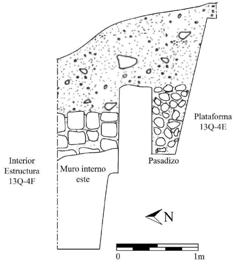
Figura 4.12 Perfil este Unidad CR20F-16 (Dibujo por E. Bustamante).
