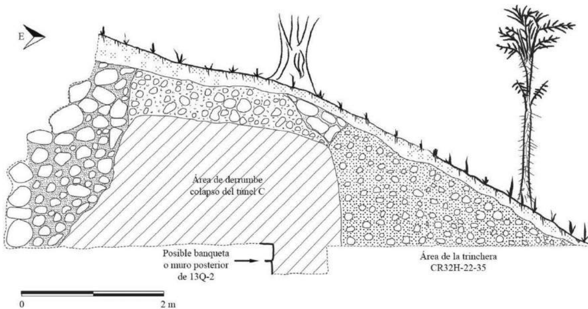
Figura 6.13 Perfil norte del extremo este del túnel C y la Unidad CR32H-22-35, mostrando la posible banqueta o muro y el sector del colapso (Dibujo por R. López).
