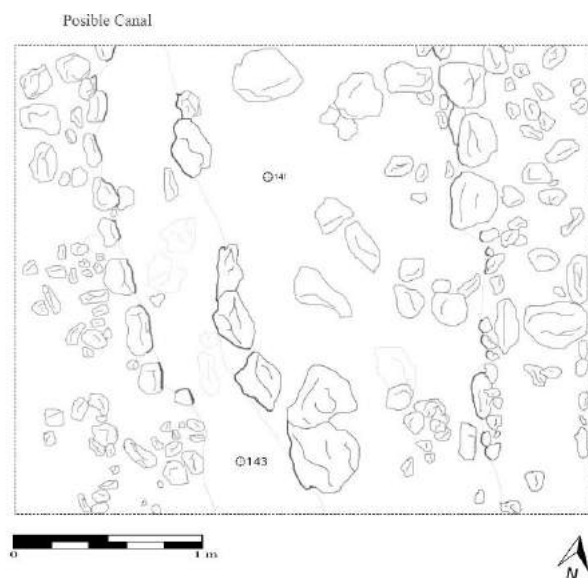
Figura 7.3 Planta de la Unidad CR52A-1. (Dibujo por M. López, digitalización por R. González).
