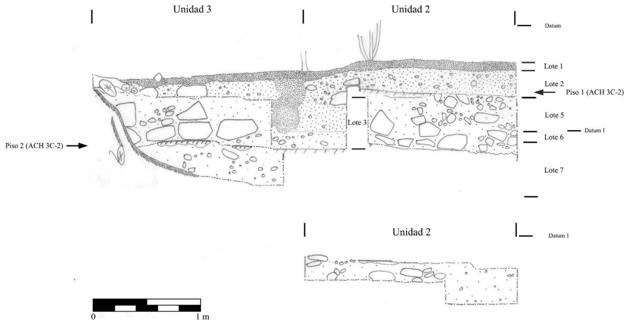
Figura 8.20 ACH 3C-2 y 3, Perfil Sur, con perfiles integrados de 2017
