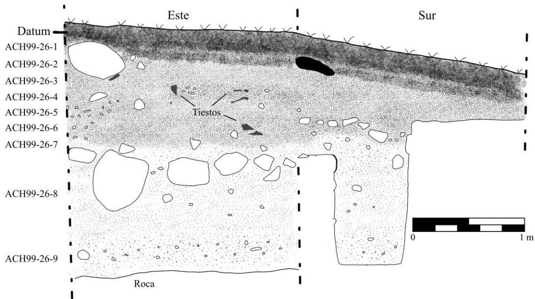
Figura 7.22 Perfiles este y sur de la Unidad ACH99-26 (Dibujo por L. Auld-Thomas)
