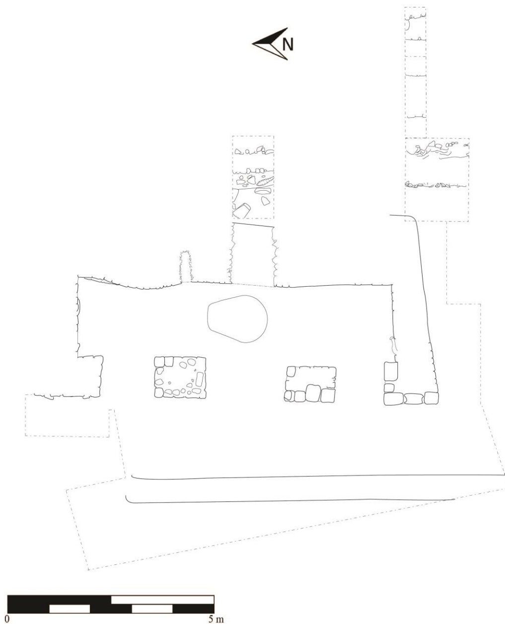
Figura 14.4 Planta de excavaciones de la Estructura 13R-45, con la ubicación del Altar 5 (Dibujo por A. Cajás, modificado y digitalizado por A. González)
